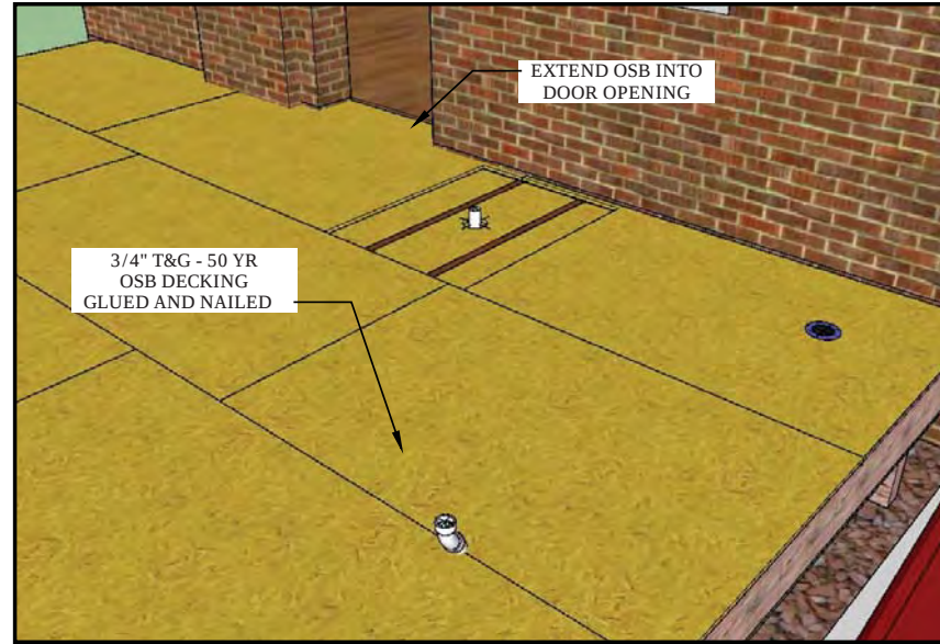
3 OSB DECKING Scale: NTS
